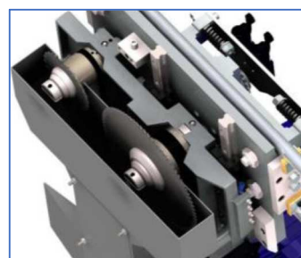
Sistema de serra e riscador da Seccionadora
